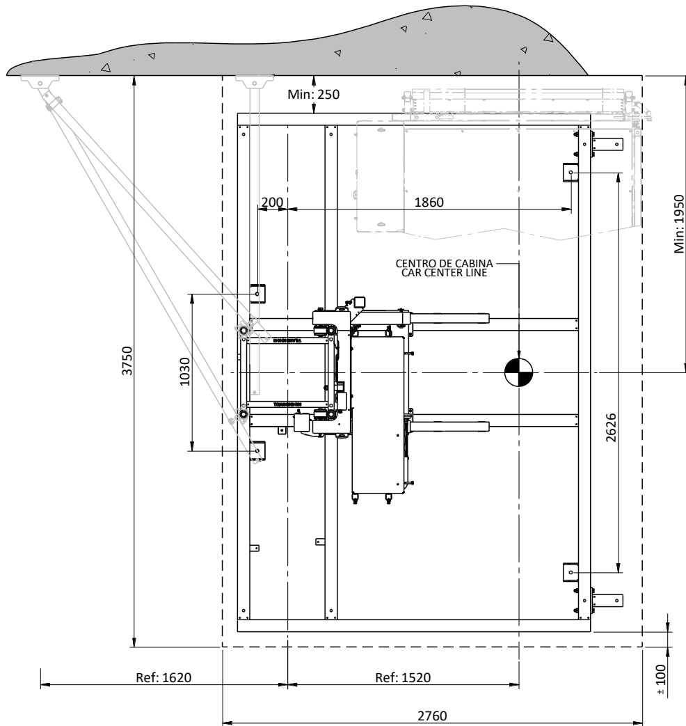
DIMENSIONES MÍNIMAS DE LA LOSA DE APOYO Y POSICIONAMIENTO BASE
