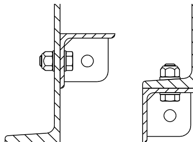
BRIDA ATORNILLADA A ESTRUCTURA METALICA
