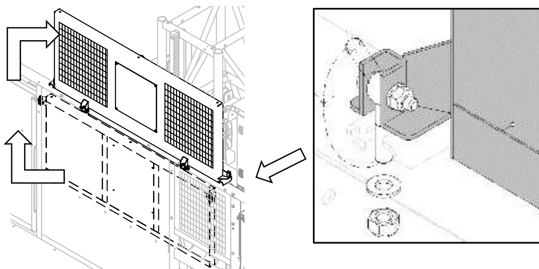
MONTAJE DEL PROTECTOR DE MASTIL
