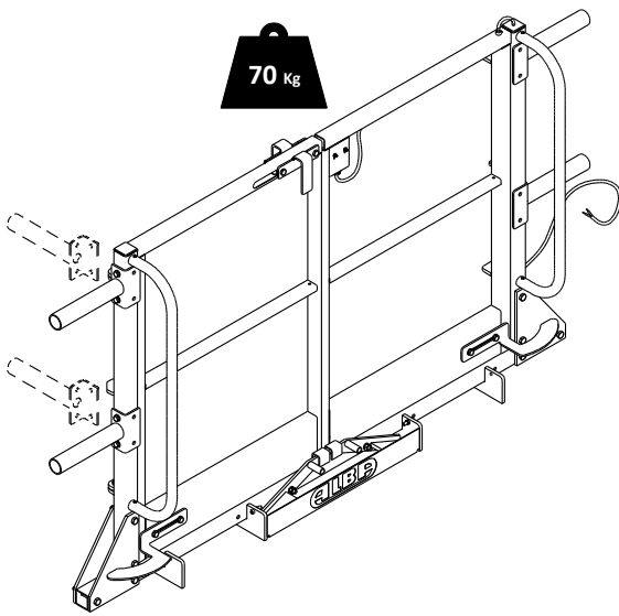
163.5 PUERTA DE PLANTA BATIENTE 1400
