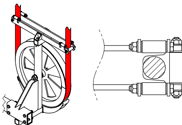
POSICION DE CABLE EN EL CARRO
