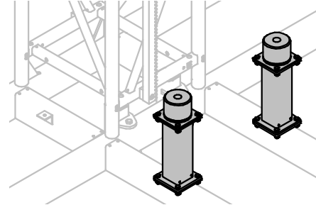
AMORTIGUADORES PARA CARRO:
