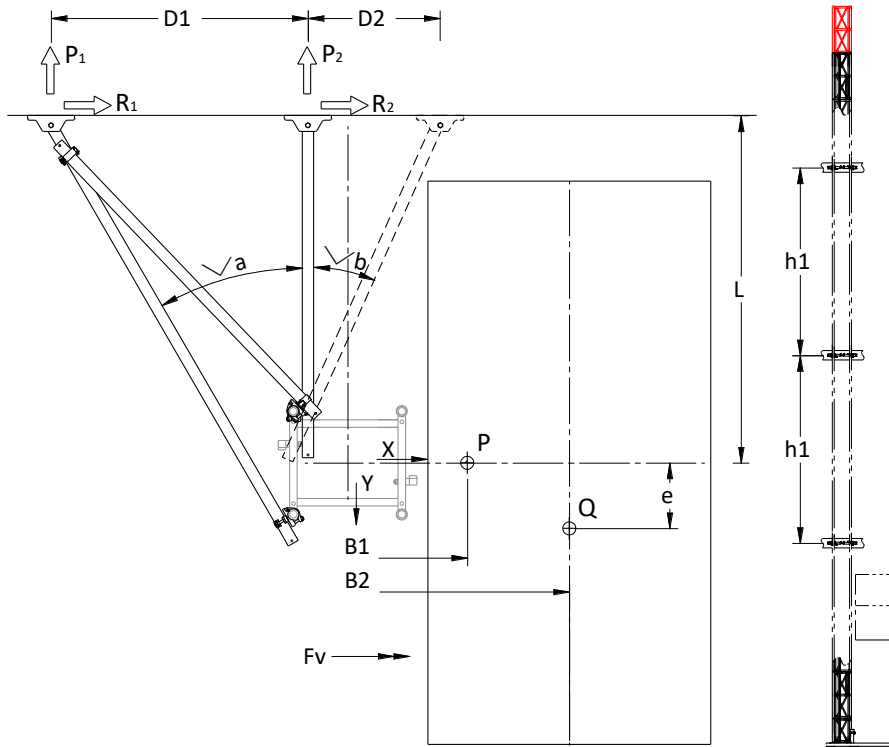
BRIDA MONTAJE SOBRE FORJADO (Ref: 153.84)
