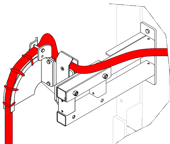
SOPORTE DE SALIDA DE CABLE EN CABINA
