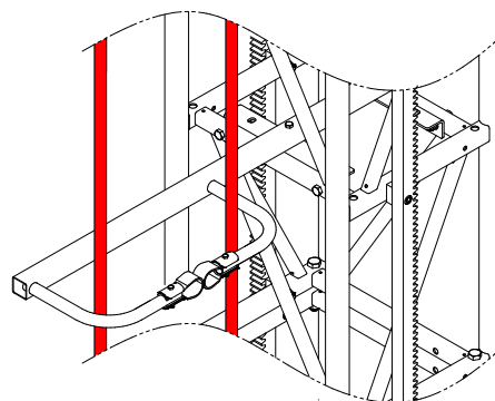
INSTALACION DE GUIAS DE CABLE
