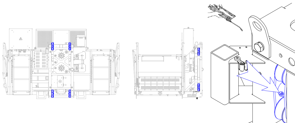
PUNTOS DE ENGRASE EN CABINA
