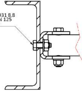
BRIDA ATORNILLADA A ESTRUCTURA METALICA
