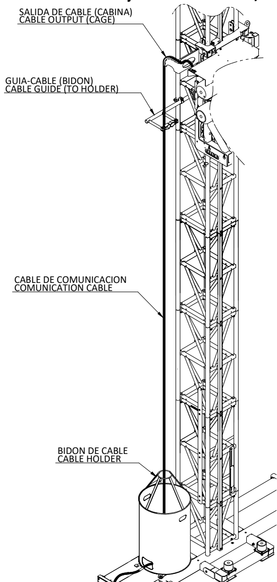
INSTALACION DEL BIDON DE CABLE
