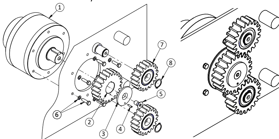
MONTAJE DEL FRENO PARACAIIDAS
