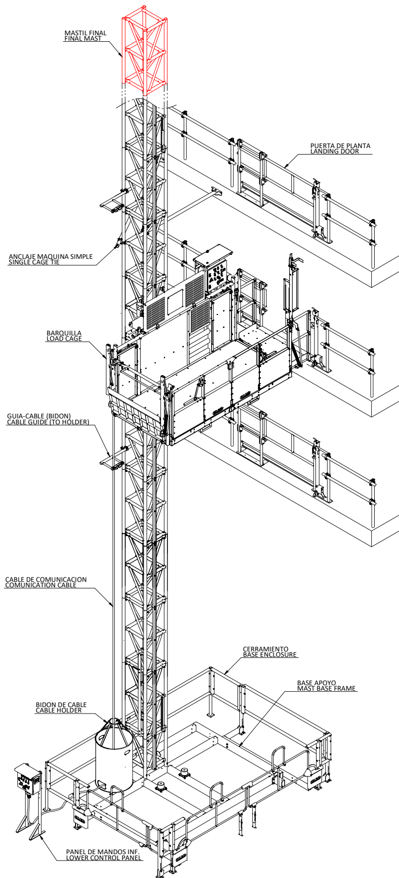
ESQUEMA DE MONTAJE MC 2000F
