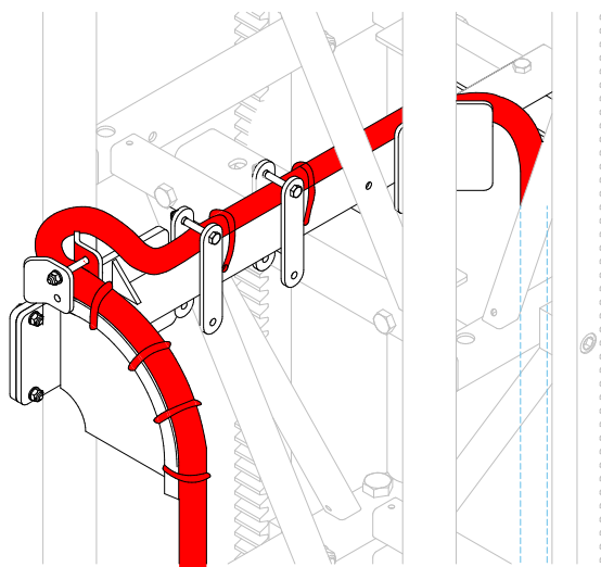
SOPORTE DE SALIDA DE CABLE DEL MASTIL
