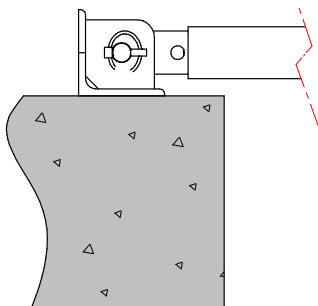
MONTAJE SOBRE / BAJO FORJADO
