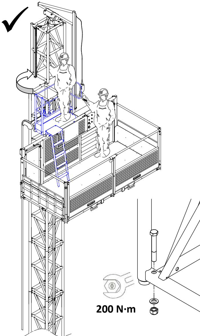
MONTAJE MANUAL DE LA COLUMNA DE MASTILES
