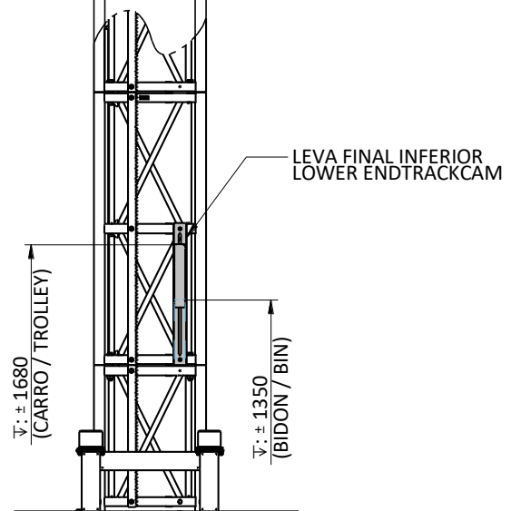
POS. LEVAS FINAL DE CARRERA Y MASTIL ROJO
