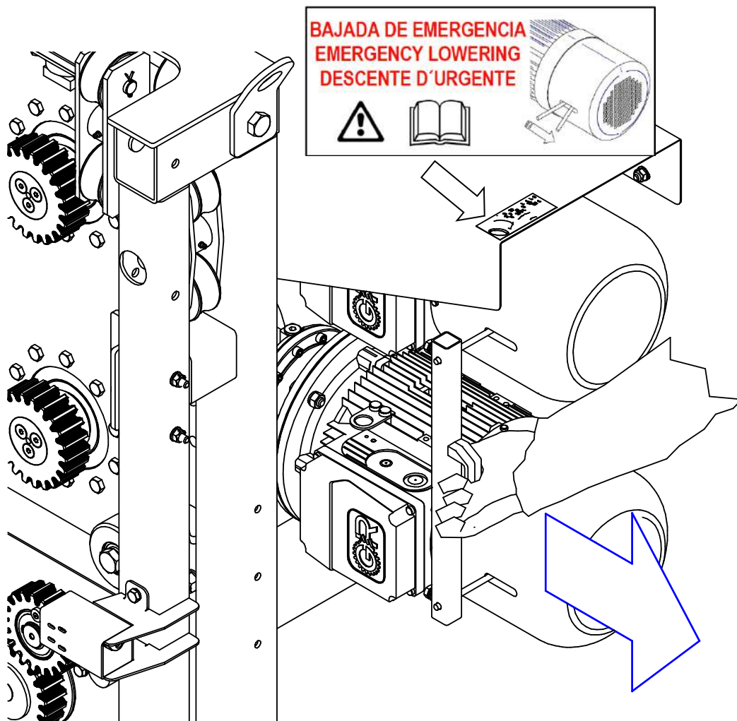
DESBLOQUEO DE FRENOS. BAJADA DE EMERGENCIA
