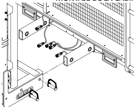
ACOPLAMIENTO DE LA CABINA
