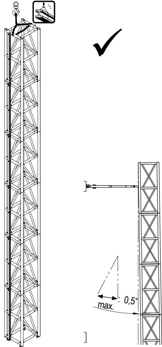
RECOMENDACION DE MONTAJE CON GRUA
