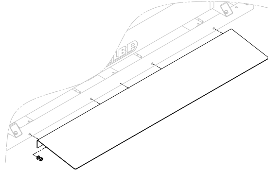
OPCIONAL – 161.56 RAMPA DE ACCESO (∠ 10°)
