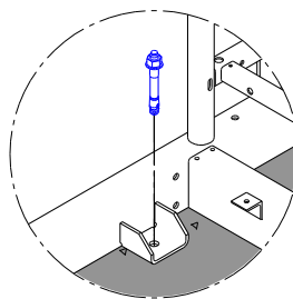
FIJACION DE LA BASE AL SUELO
