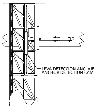
ZONA TRASERA MASTIL
