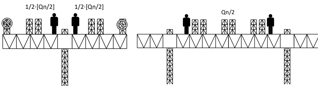
CARGA DE LA PLATAFORMA DURANTE EL MONTAJE MÁSTILES
