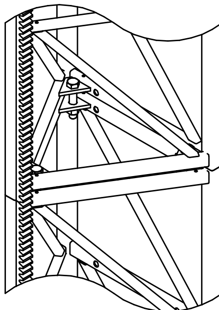
MONTAJE DE TORNILLOS DE MÁSTIL
