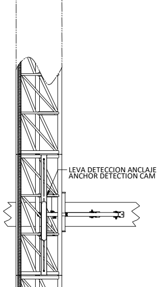
LEVAS ANCLAJE 086.392
