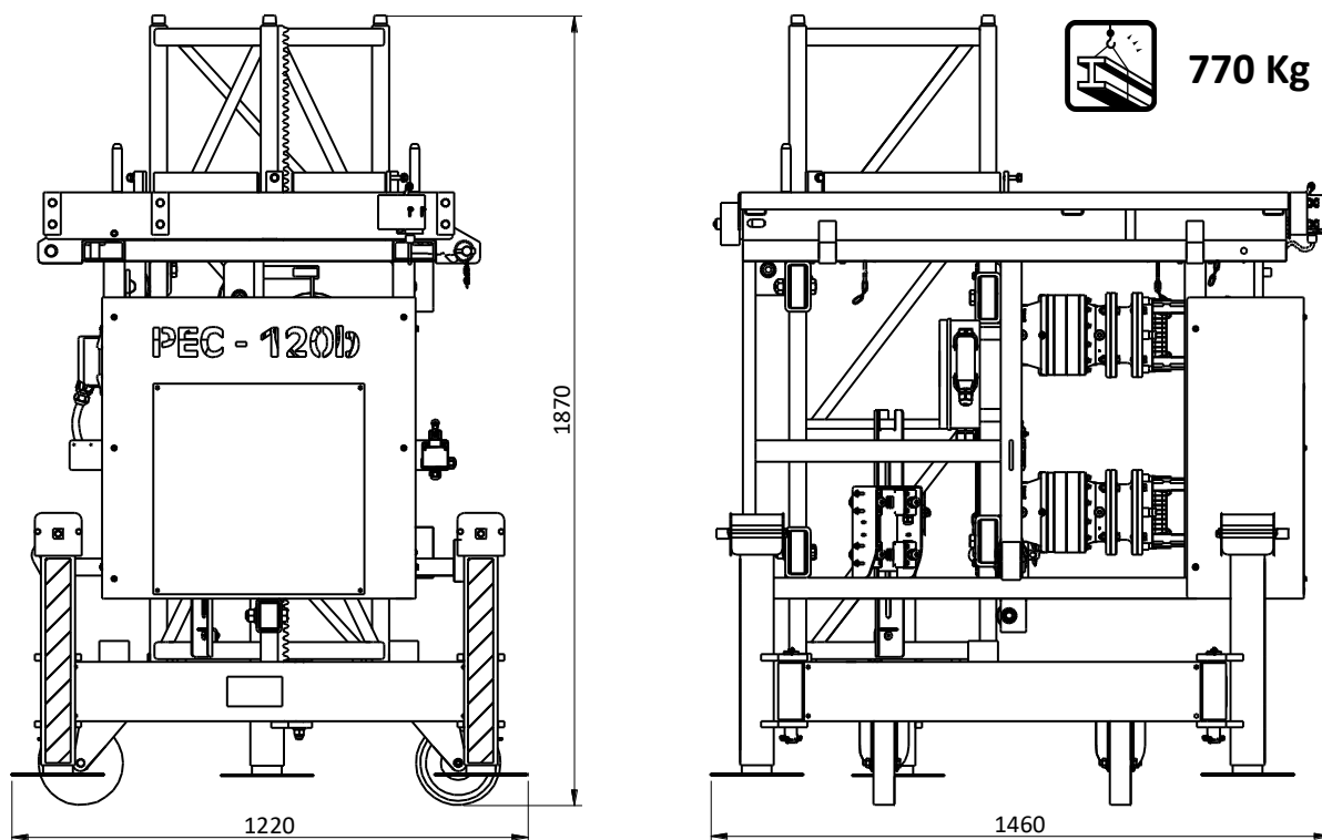
CONJUNTO BASE (EXPEDICIONES)
