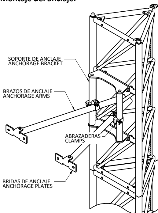
MONTAJE DEL SOPORTE DE ANCLAJE
