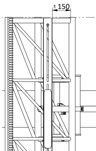
REGULACION LEVA ANCLAJE
