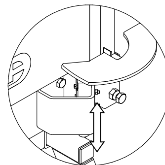
AJUSTE MICRO PUERTA
