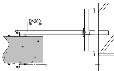
FIJACION SUPERIOR / INFERIOR
