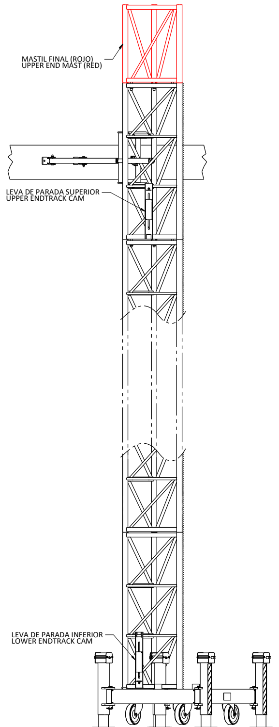
MONTAJE DE LEVAS DE PARADA
