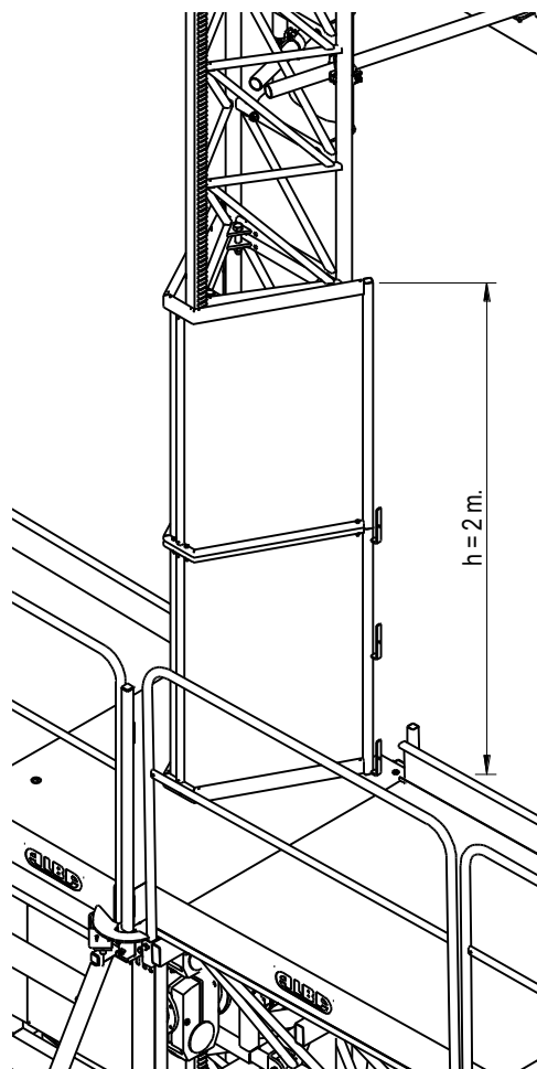
PROTECTOR DE MASTIL
