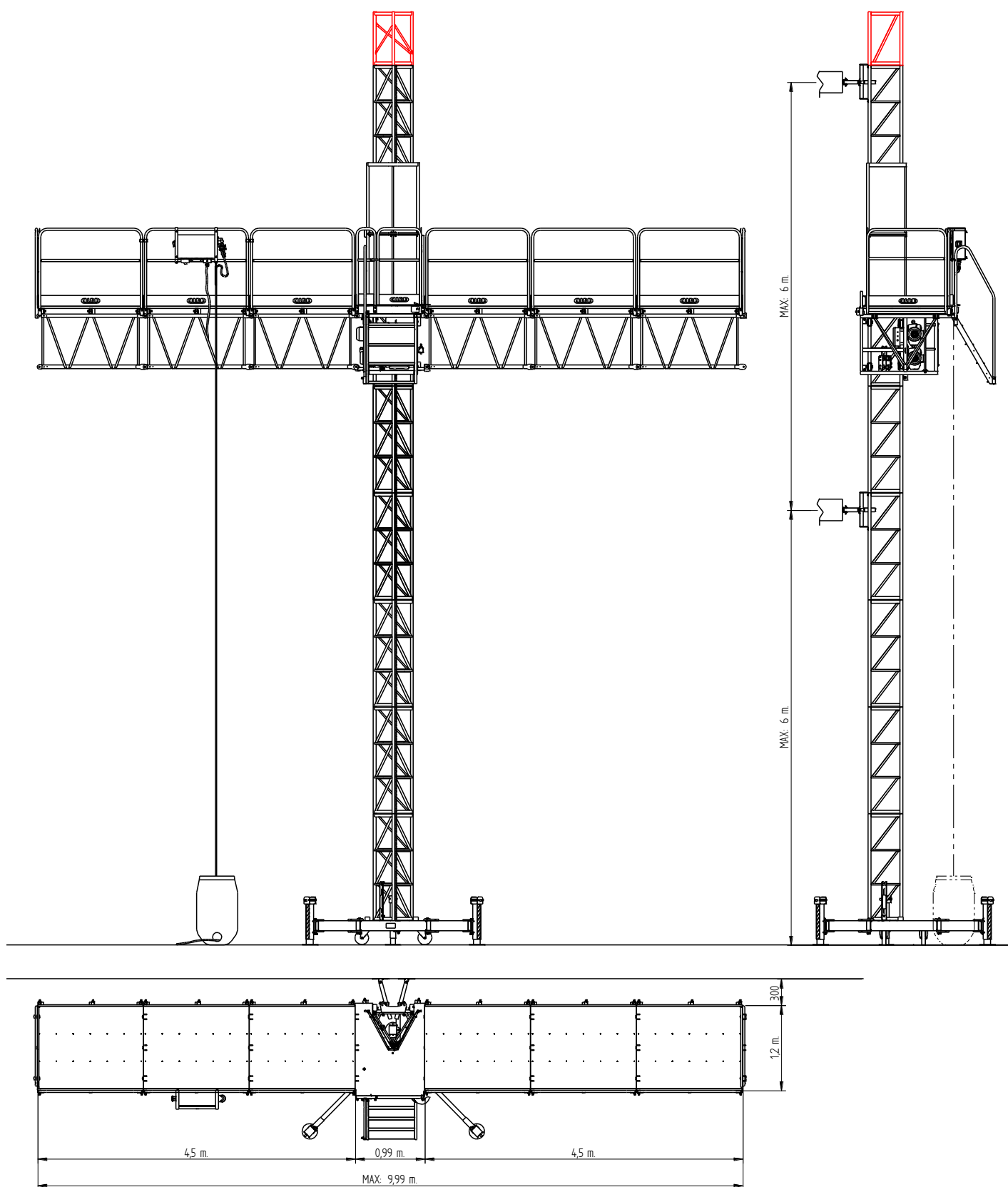
PLATAFORMA MONOMÁSTIL
