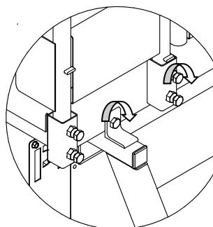
FIJACION ESCALERA Y PUERTA
