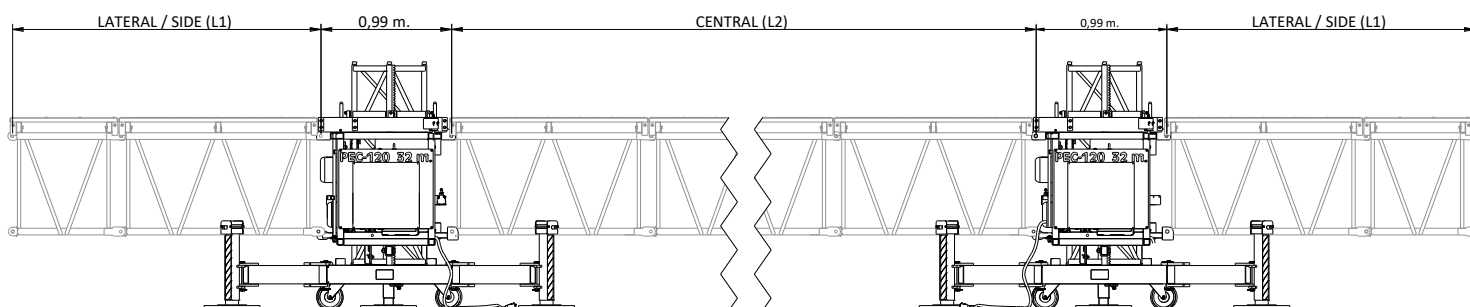
DISTRIBUCIÓN FINAL DE PLATAFORMAS BIMASTIL
