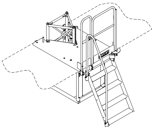
MONTAJE DE PUERTA Y ESCALERA
