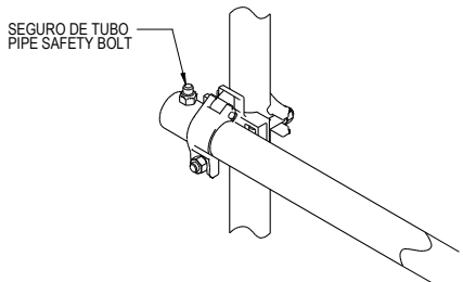
A TUBOS VERTICALES / ANDAMIO
