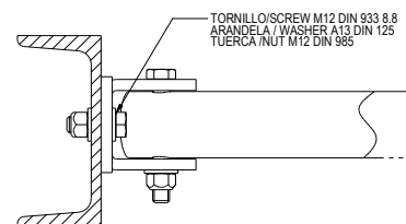
FIJACION ATORNILLADA
