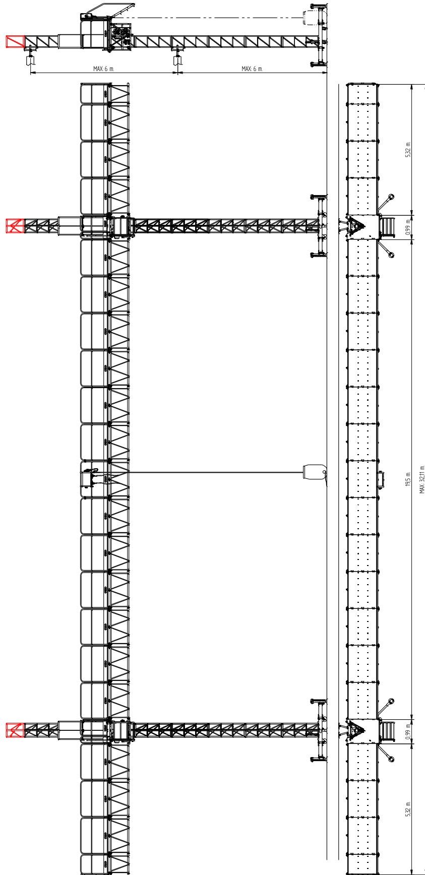
PLATAFORMA BIMÁSTIL
