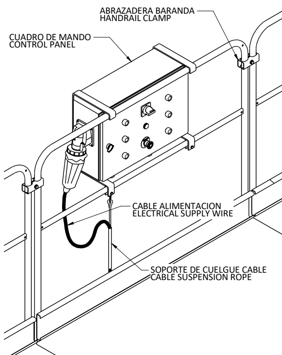
MONTAJE CUADRO DE MANIOBRA
