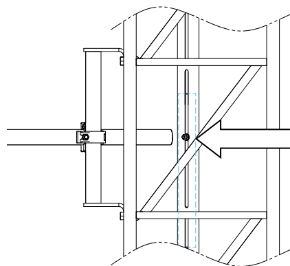
ZONA TRASERA MASTIL
