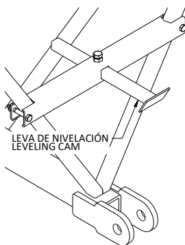
MONTAJE LEVA
