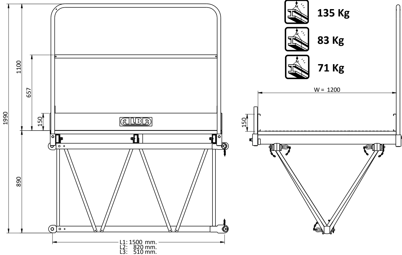
CONJUNTO PLATAFORMA
