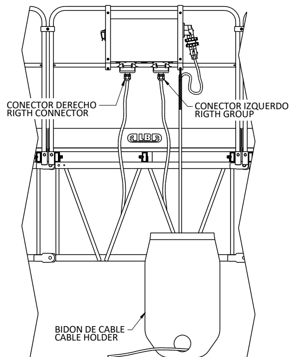
MONTAJE BIDÓN DE CABLE
