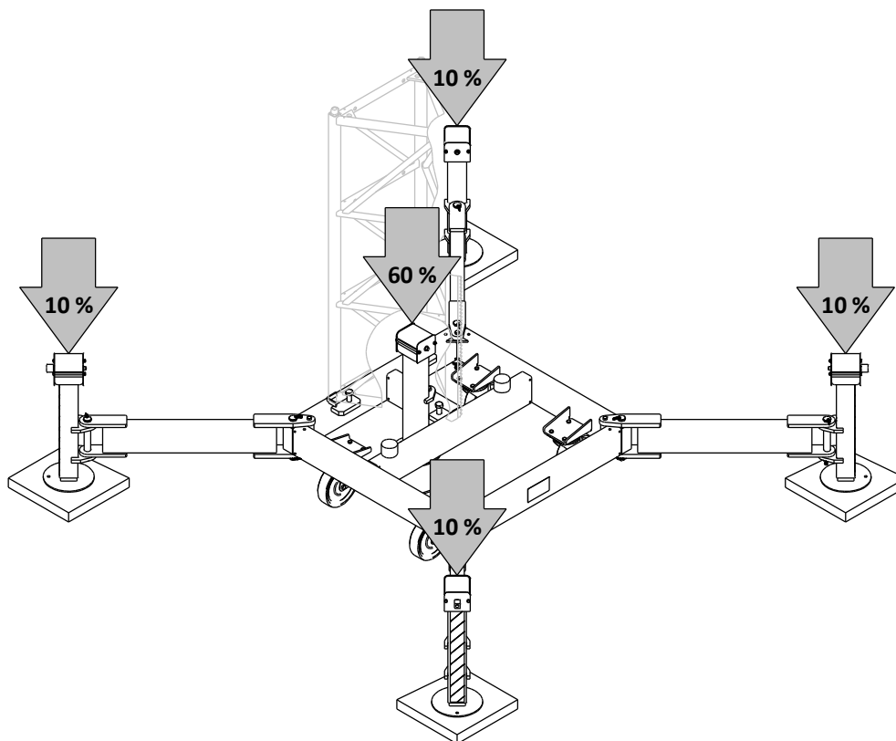
DISTRIBUCIÓN DE CARGAS A LOS APOYOS
